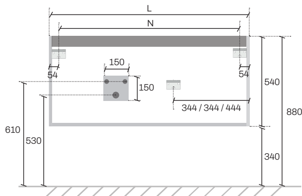
Lavabo izquierda Vasque gauche / Left basin
