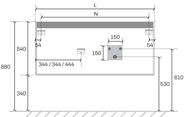
Lavabo derecha Vasque droite / Right basin
